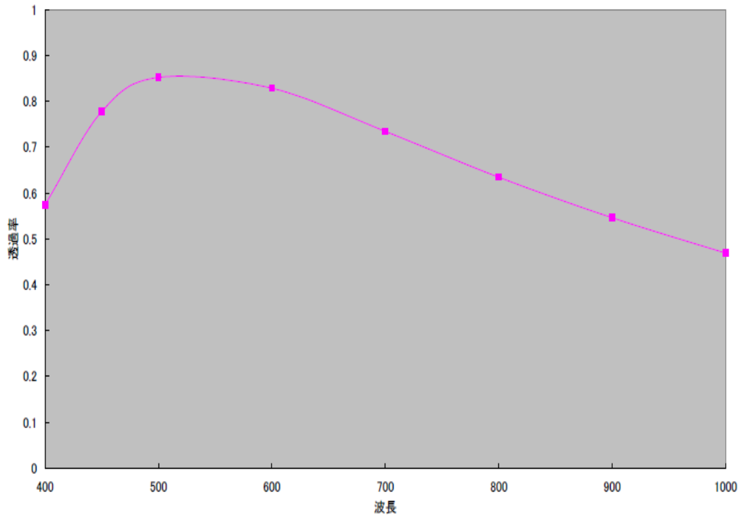
LMVZ3510 (1030) 透過率
